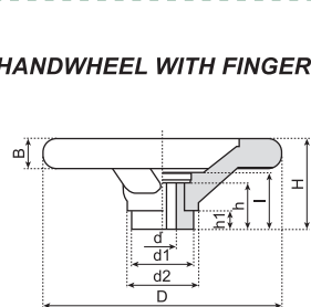
A 型 (TYPE A)
