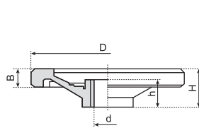
A 型 (TYPE A)
