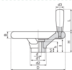
B 型 (TYPE B)
