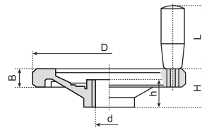
B 型 (TYPE B)
